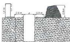
"A" és "B" méretel SZ 219 szerinti A = 0,6 m ; B = 1,0 m Hogaszálási (szjuk) (has) = min. 1,5 x 1,0 m
