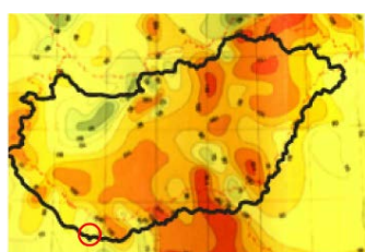
1.16-17. ábra: Magyarország geotermikus energiahordozó hasznosítási lehetősége – A Pannon- medencének és régiójának geotermikus hőtérképe (részlet) Forrás: PannErgy, Portfolio.hu
